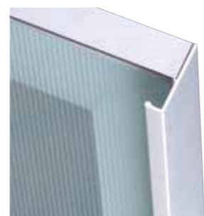
H5 גלאס גריפ ללא כרסום ידית לפרופילי אלומיניום. גימור: טבעי.
