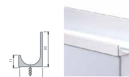
H15 מידי קעור מתאים לדלתות: ציפורי, אולטרא גלוס, עדן C2, C3, C5, בניאס, אלומקס - גלקסי, נגה. גימור הידיית: טבעי/ברק משי/צבע.
