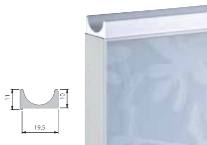
H14 מיני קעור ידית לפרופילי אלומיניום. גימור: טבעי.
