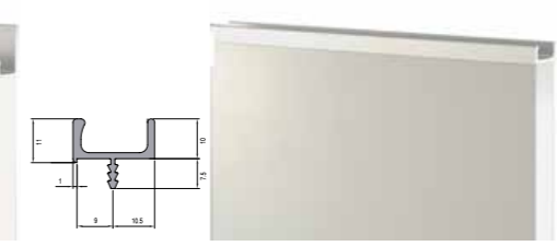
H23 מיני טרפז מתאים לדלתות: ציפורי, אולטרה גלוס, בניאס. גימור הידית: טבעי/צבע.
