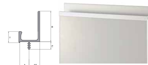
H24 מידי טרפז מתאים לדלתות: ציפורי, אולטרה גלוס, בניאס. גימור הידית: טבעי/צבע.
